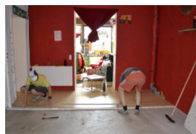
灰色のコンクリートの床も悪くはなかったが、やはり木製の床には敵わない! 地階からの冷気を防ぐため、発泡スチロールの板を間に敷いた。
